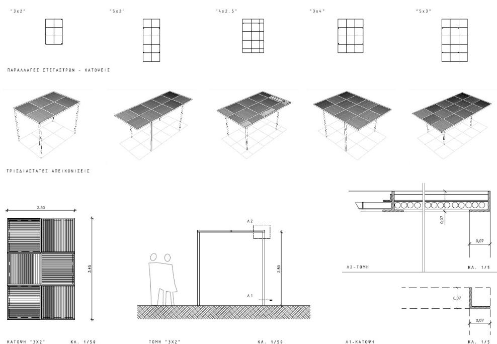
Εικόνα 27 Τυπολογία στεγάστρων ανάλογα με το σημείο στάσης
