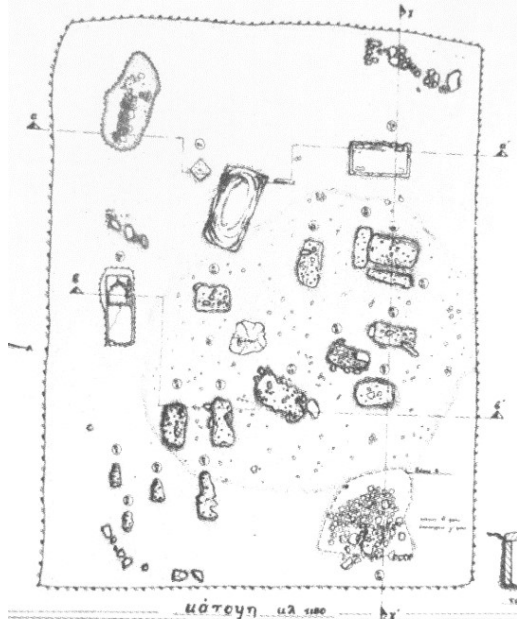
Εικόνα 4 Κάτοψη νεκροταφείου κλασικών χρόνων (θ.15) (Από το αρχείο της ΕΦΑΑΝΑΤ).
