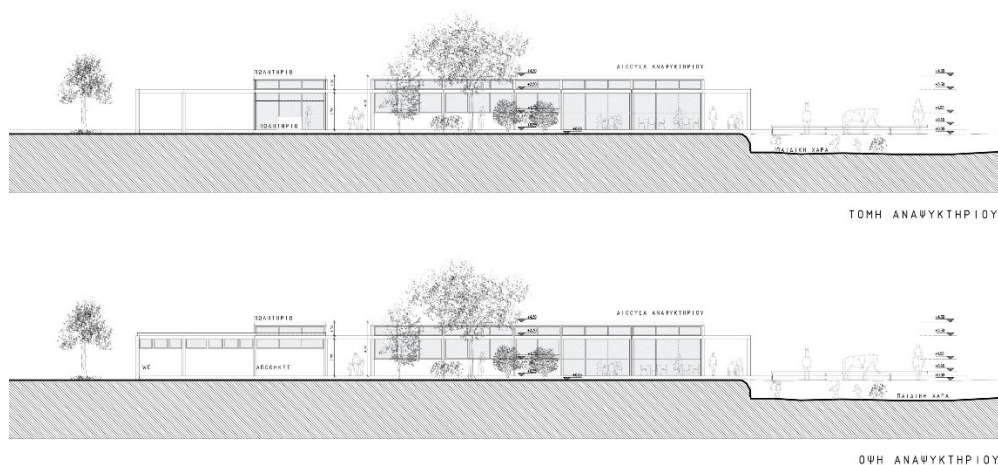
Εικόνα 25 Σχέδια όψεων και τομών του αναψυκτήριου και του πωλητηρίου
