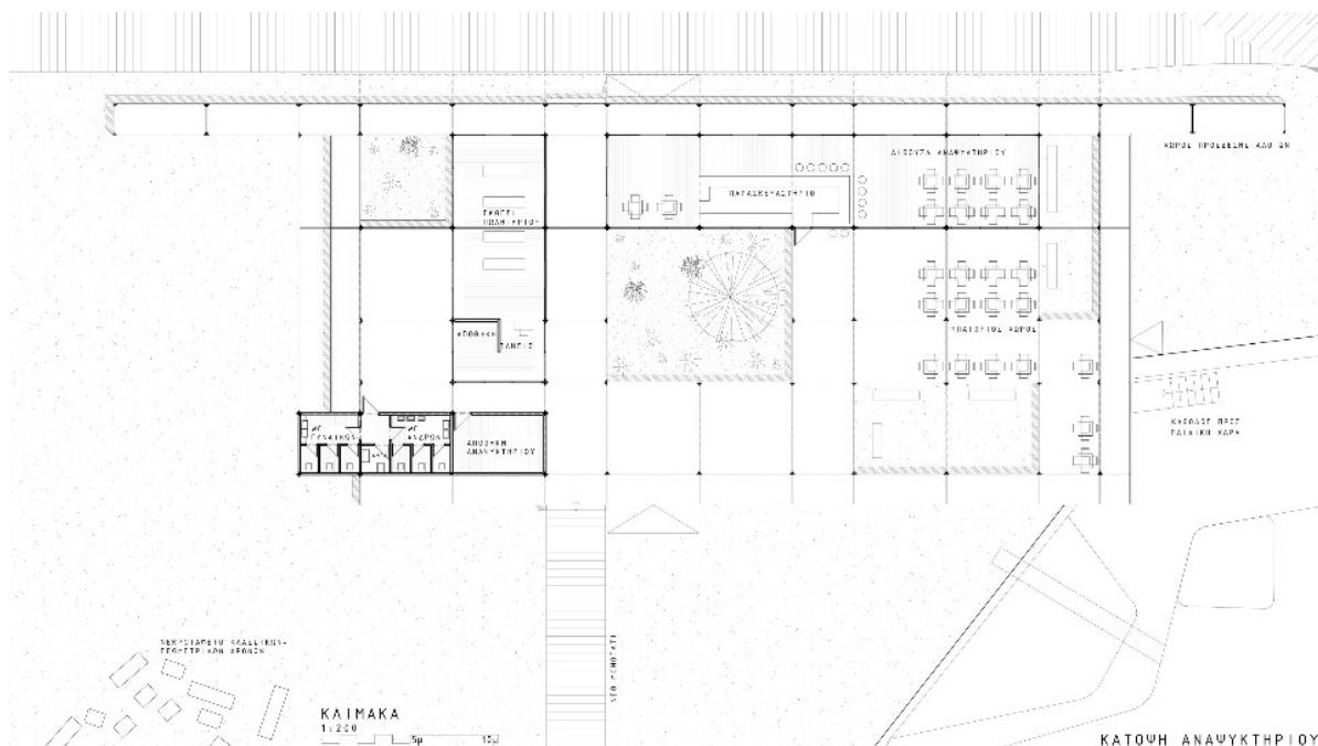
Εικόνα 23 Σχέδιο κάτοψης του αναψυκτήριου και του πωλητηρίου
