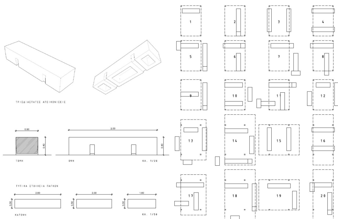
Εικόνα 28 Μπετονένιοι πάγκοι και τυπολογία διάταξης καθιστικών
